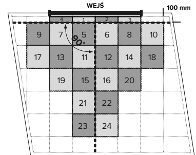
Instalacja Fortelock LIGHT, INDUSTRY, XL
