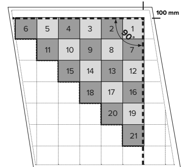
Instalacja Fortelock DECOR, INVISIBLE
